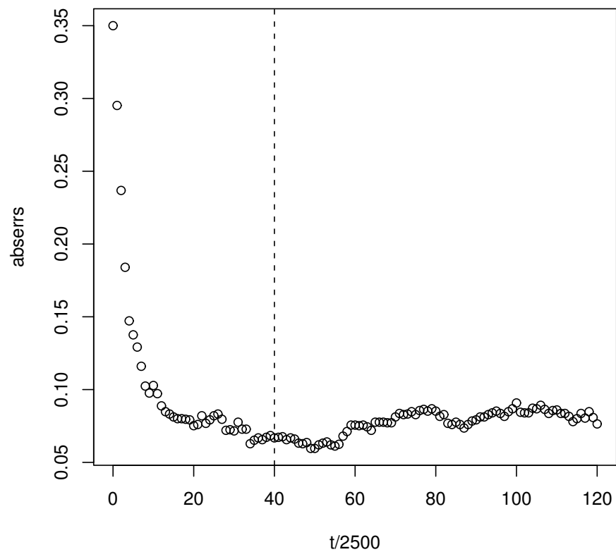
図 17 (左) 真の画像からの誤差 \sum_i |X_t[i] - x[i]| / (2m^2) の値 , (右) 定数項を無視した \log f(\mathbf{X}_t | \mathbf{y}) の値 , つまり式 (1.8) の右辺にある exp 関数の引数の値
