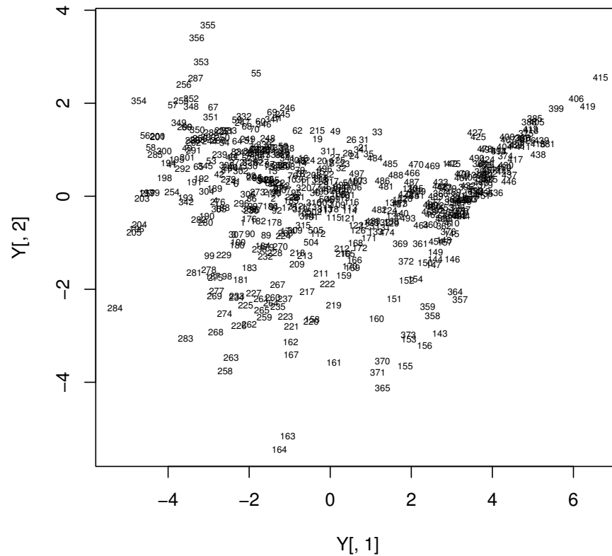
図 31 ポストン住宅価格データの主成分 . (左) 第 1 主成分から第 14 主成分までのペア毎の散布図 . (右) 第 1 と第 2 主成分のプロット .
