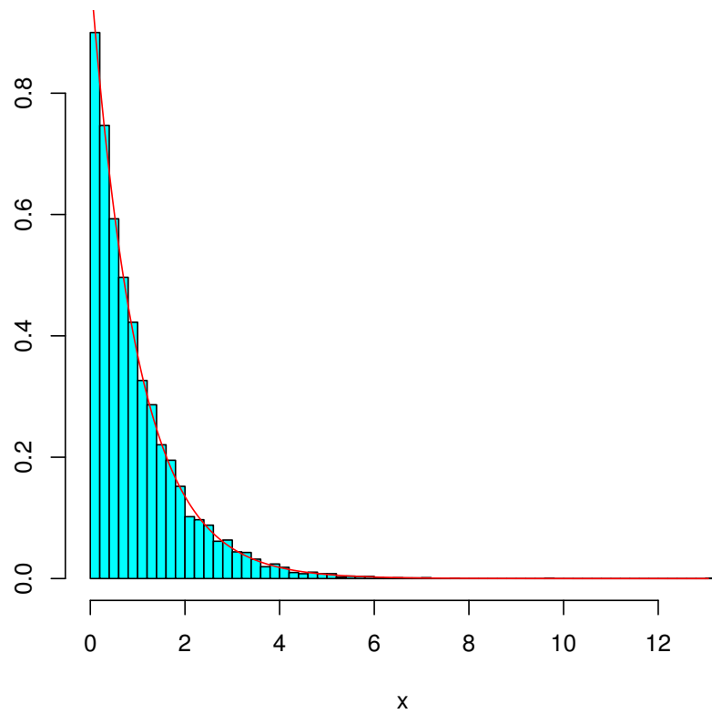
图 10 (左) 逆関数法 (指数分布), (右) 棄却法 (正規分布)
