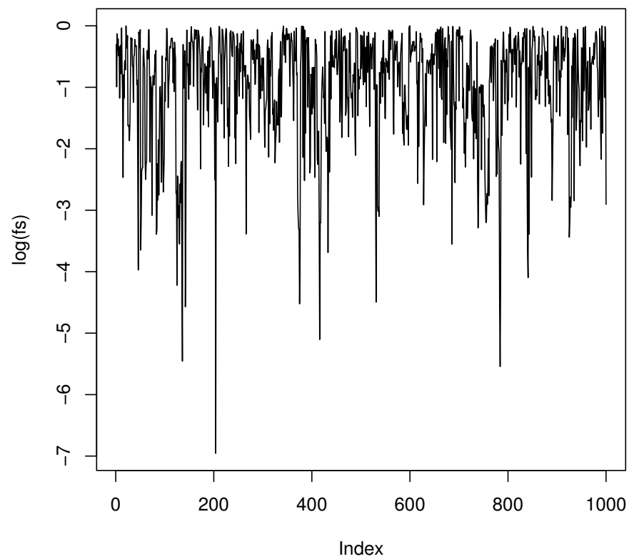
図 13 (左) 例題 1.12 の X_t , (右) \log(f(X_t))
