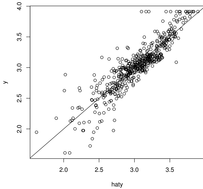
図 26 (左) (\hat{y}_t, y_t) のプロット , (右) (\hat{y}_t, e_t) のプロット
