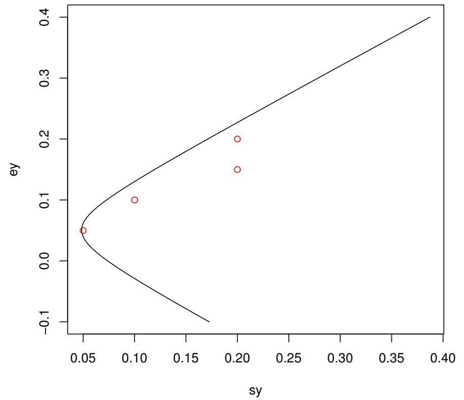
図5 (左) 独立な場合, (右) 平均-標準偏差ダイアグラム
