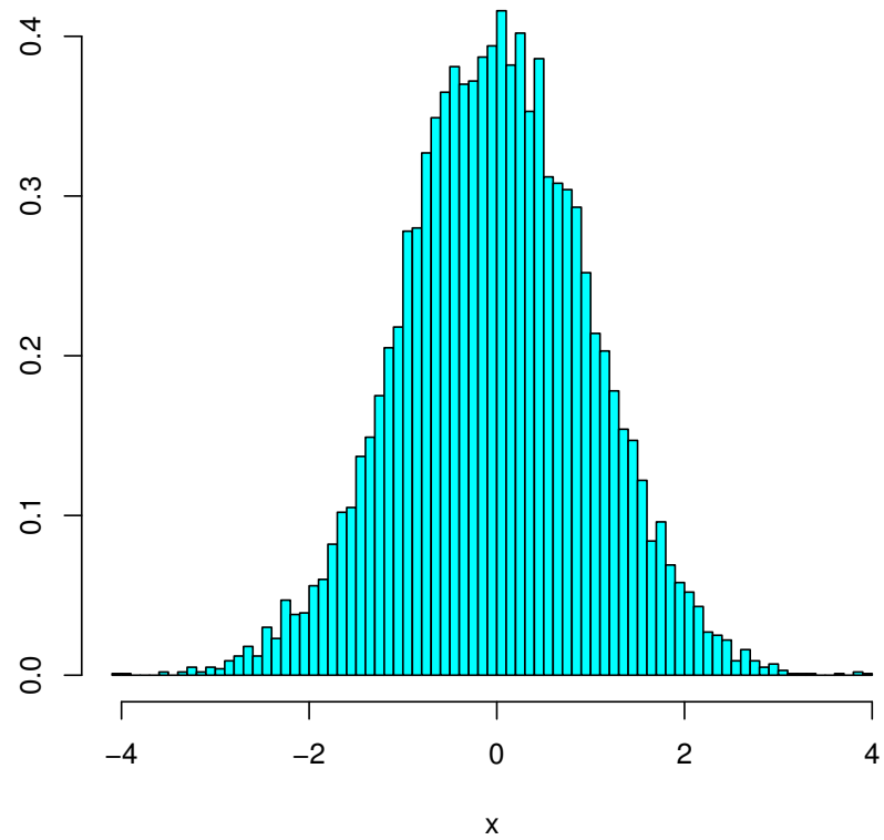
図9 (左) デフォルトの2倍の区間数 ,(右) 半分の区間数
