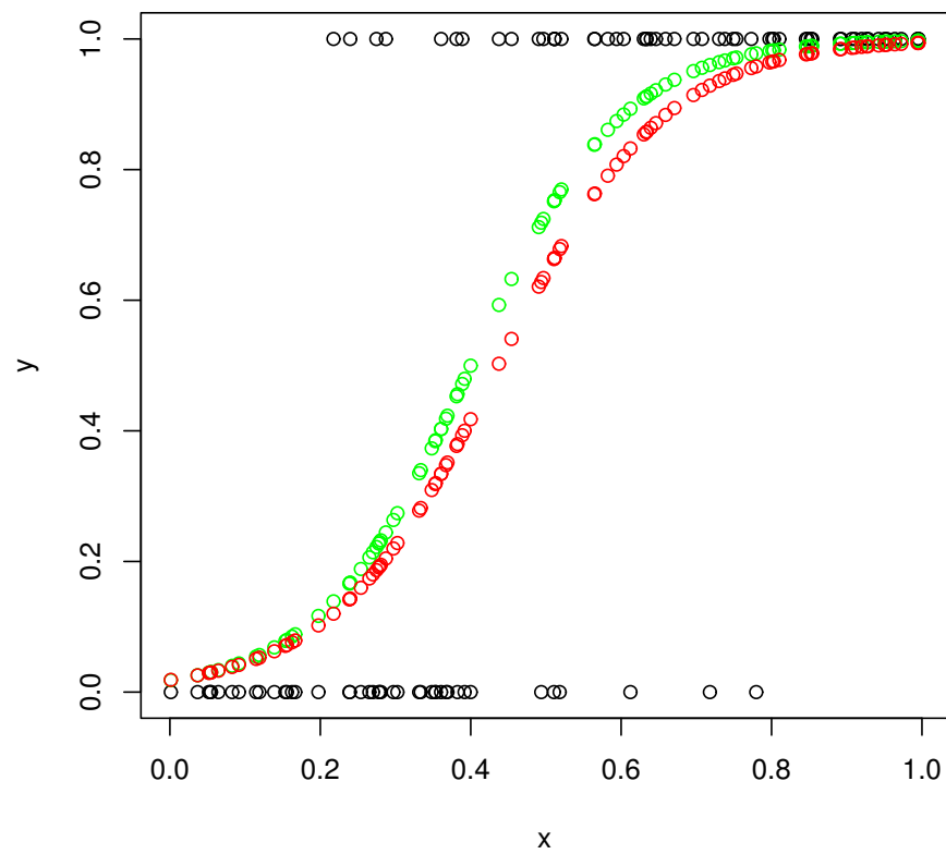
図 28 (左) ロジスティック関数 , (右) \beta = (-4, 10) から生成した (x_t, y_t)
