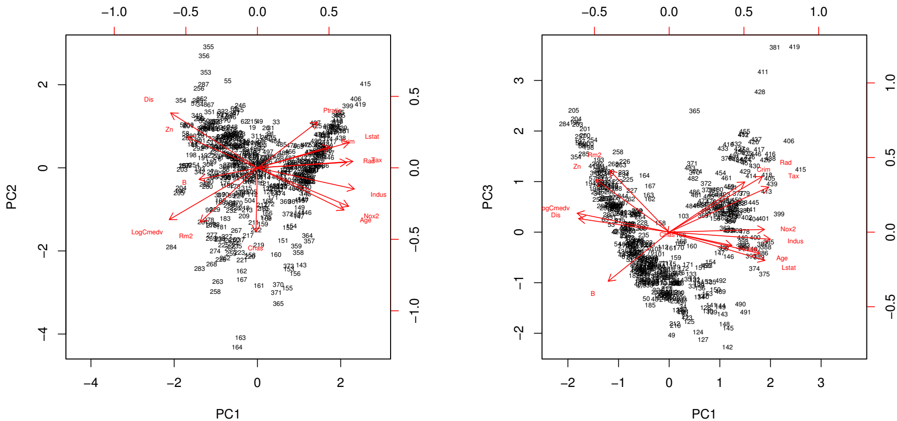
図 32 ボストン住宅価格データのバイプロット
