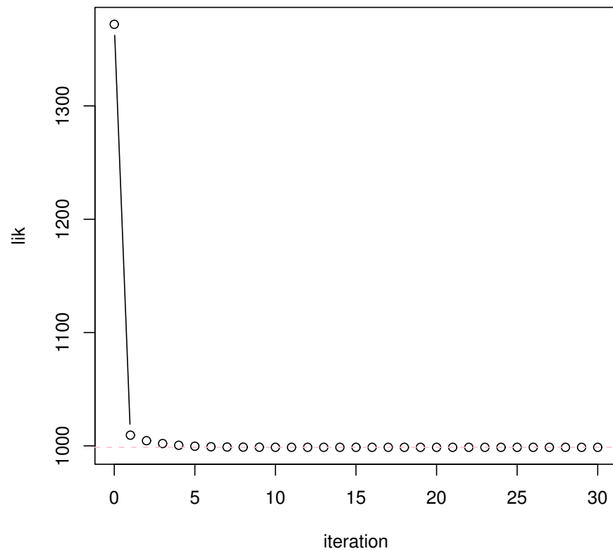
図 24 (左) -\log L(\boldsymbol{\theta}^{(r)}|\mathcal{X}_1, \mathcal{X}_2) , r = 0, \dots, 30 のプロット . 実用的には最初の 10 回程度の反復で収束した . optim による値はピンクの線で示した . (右) パラメタ \boldsymbol{\theta}^{(r)} = (\pi_1^{(r)}, \pi_2^{(r)}, \mu_1^{(r)}, \mu_2^{(r)}, \mu_3^{(r)}, \sigma_1^2{}^{(r)}, \sigma_2^2{}^{(r)}, \sigma_3^2{}^{(r)}) のプロット
