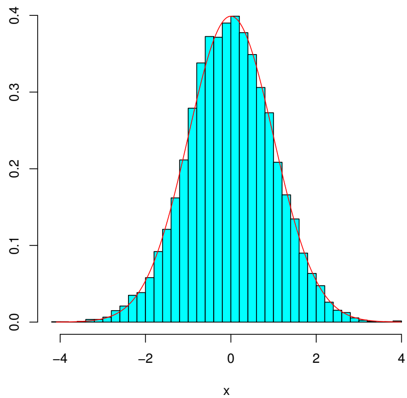
図8 (左) ヒストグラム, (右) 経験分布関数
