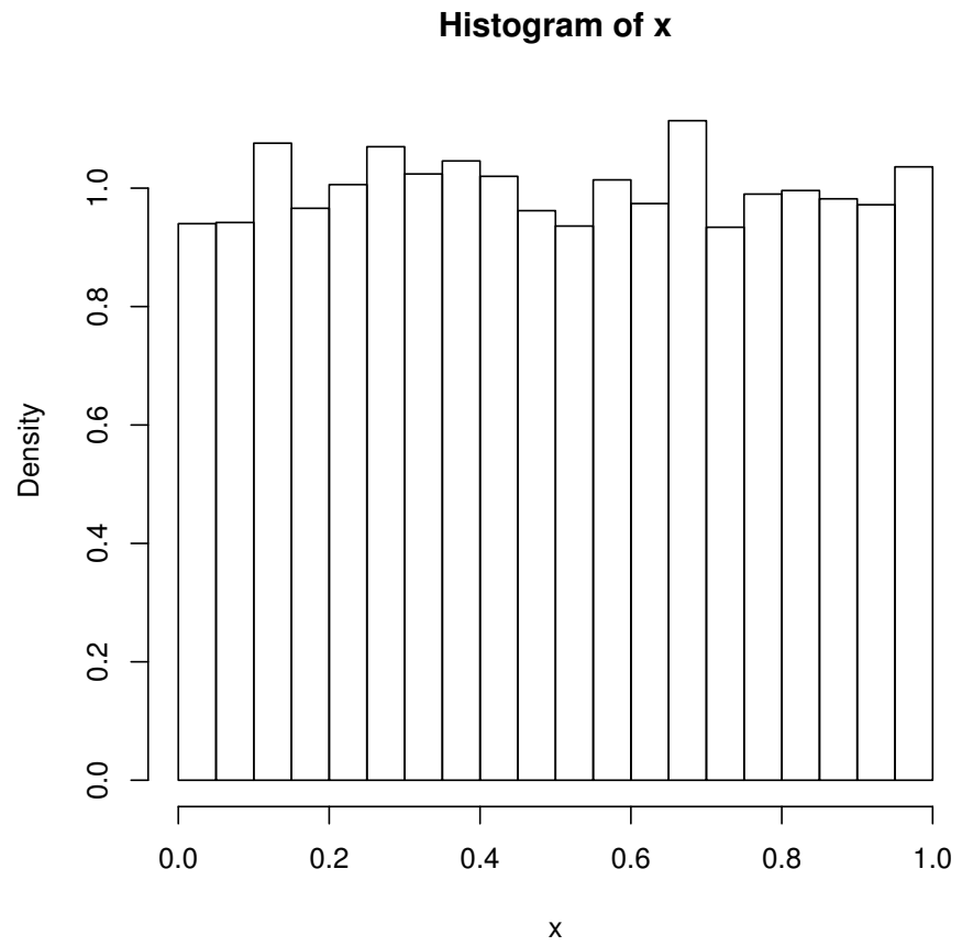
図7 (左) ヒストグラム , (右) 経験分布関数
