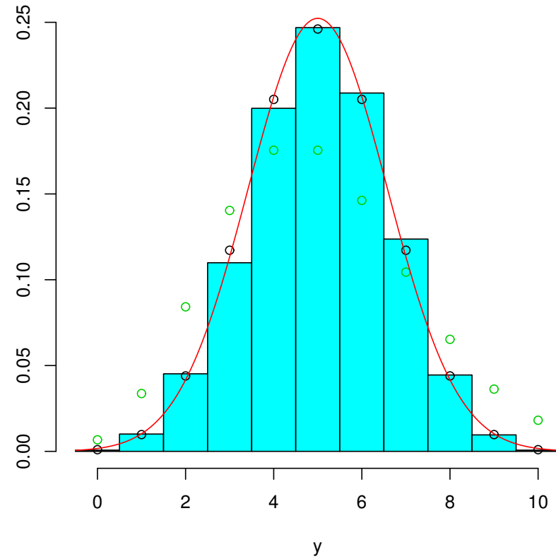
図 20 n 回のベルヌーイ試行の成功回数 . (左) n = 10, p = 0.05 では正規近似は良くない , (右) n = 10, p = 0.5 では正規近似が良い .
