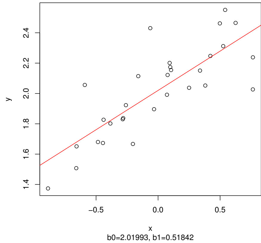
図 25 (左) データの生成, (右) 推定した回帰直線
