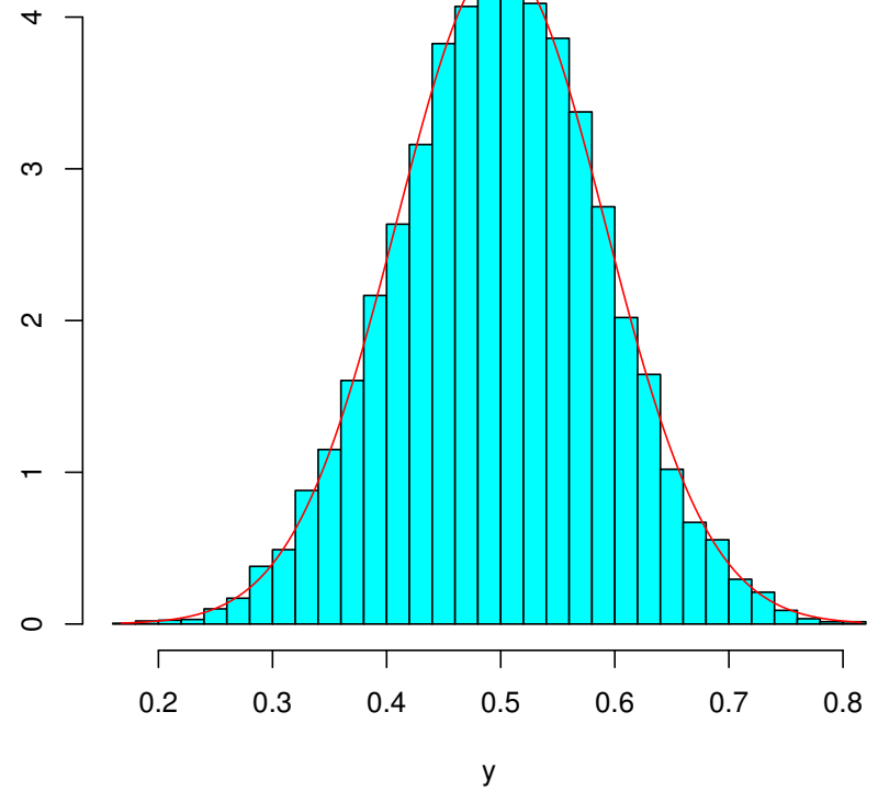
図 19 n 個の一樣分布の平均 . (左) n = 5 では正規近似は良くない , (右) n = 10 では正規近似が良い .
