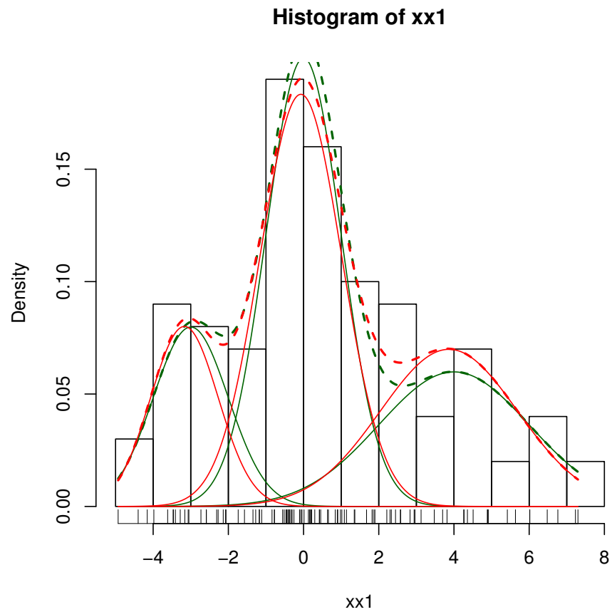
図 21 正規混合分布から生成したデータ . 真の密度関数 ( 緑 ), (x_t, i_t), t = 1, \dots, n_1 から推定した密度関数 ( 赤 ).
