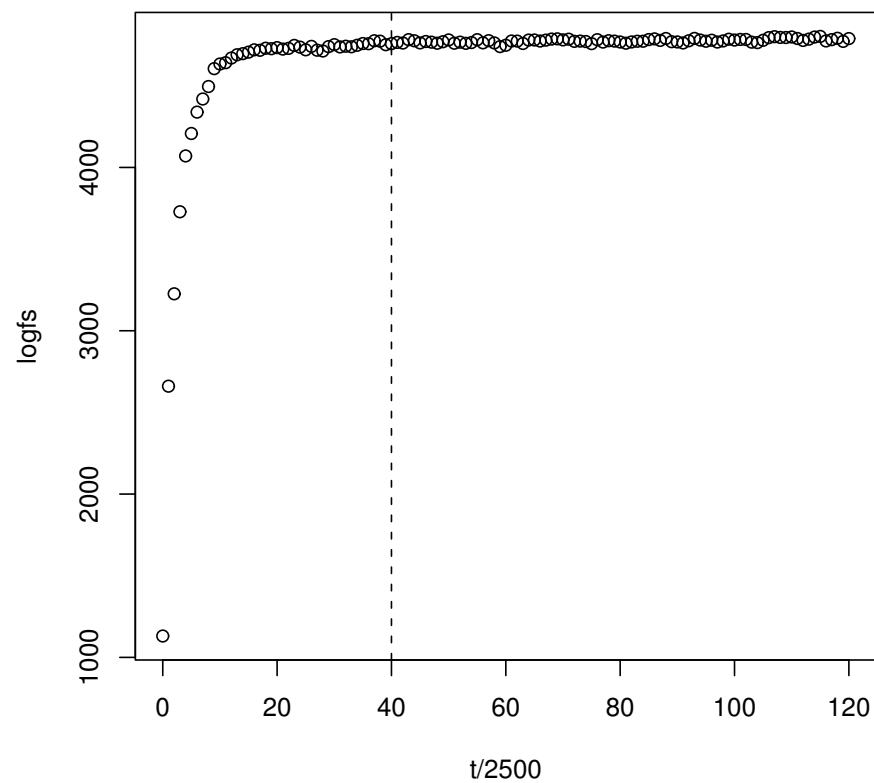
図 17 (左) 真の画像からの誤差 \sum_i |X_t[i] - x[i]| / (2m^2) の値 , (右) 定数項を無視した \log f(X_t | y) の値 , つまり式 (1.8) の右辺にある exp 関数の引数の値
