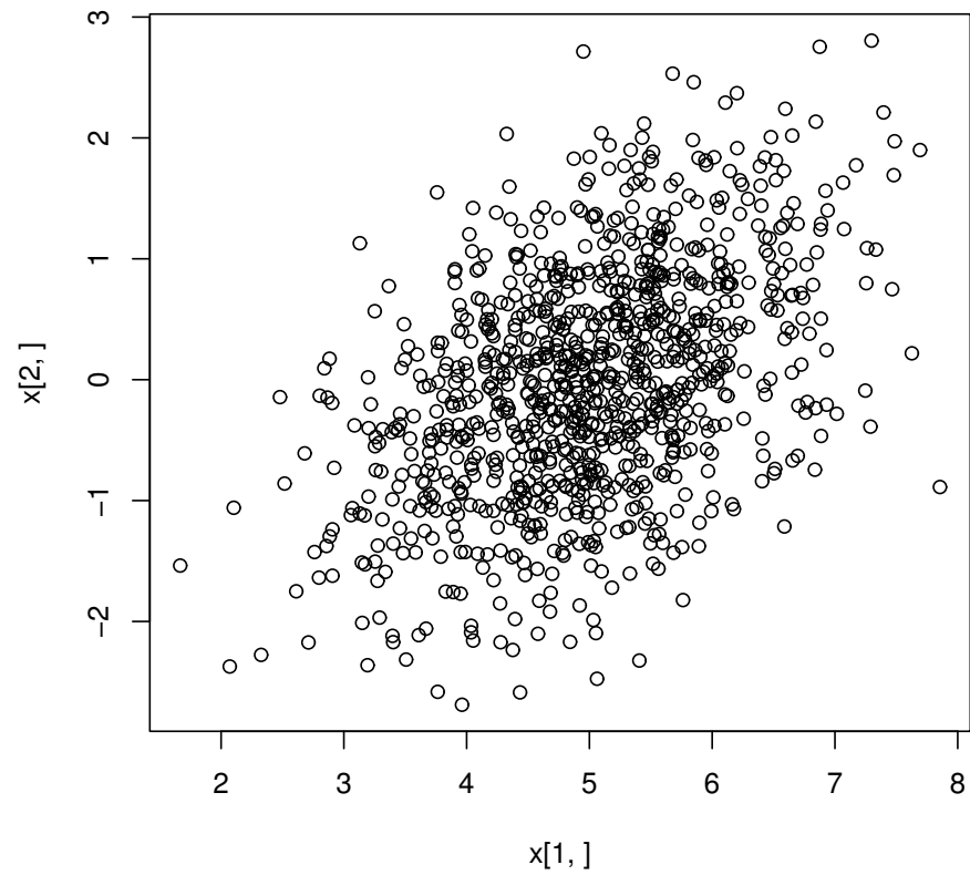
図 11 (左) 1000 個の z , (右) 1000 個の x
