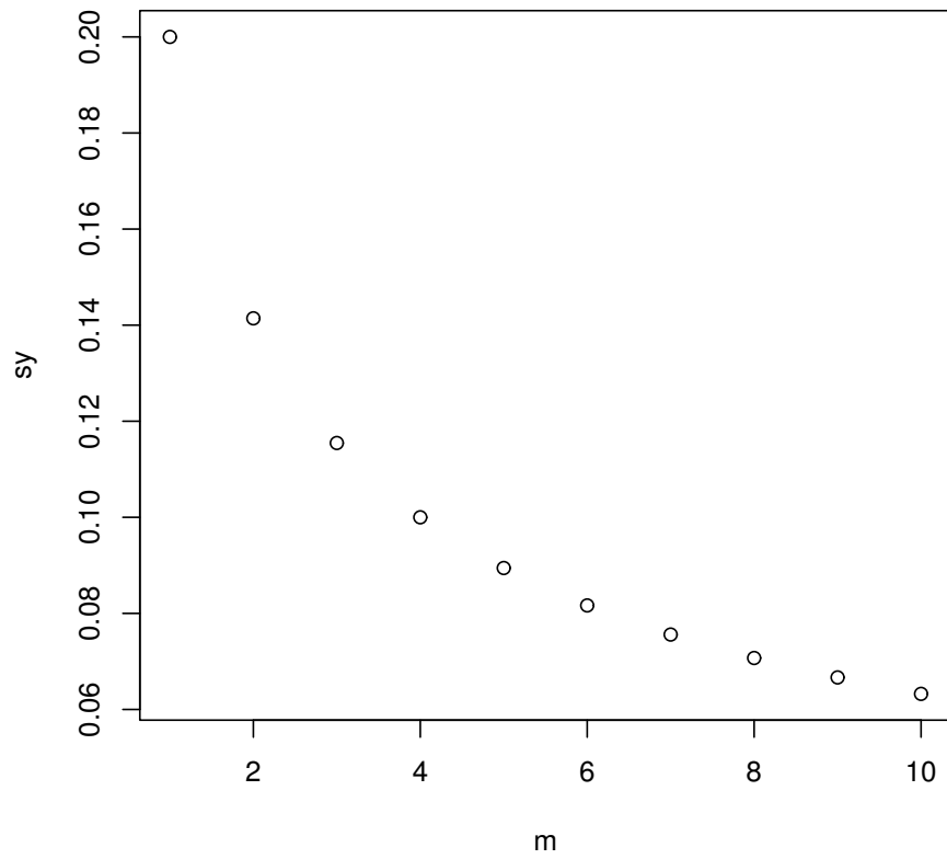
図5 (左) 独立な場合, (右) 平均-標準偏差ダイアグラム
