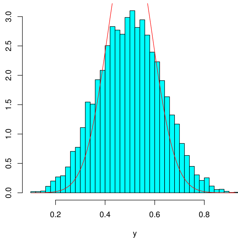
図 19 n 個の一樣分布の平均 . (左) n = 5 では正規近似は良くない , (右) n = 10 では正規近似が良い .
