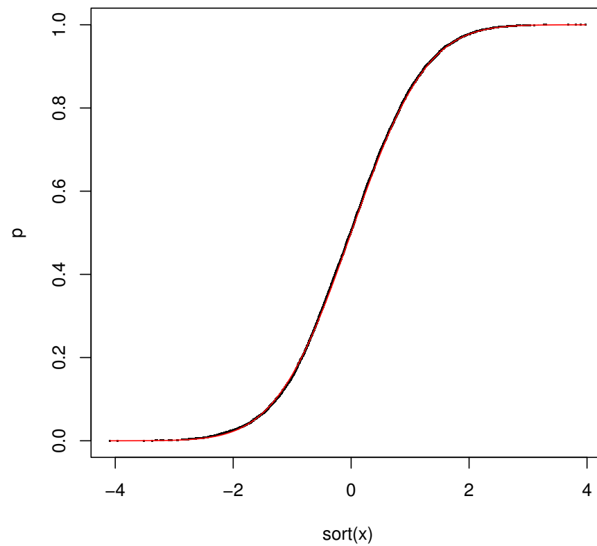
図8 (左) ヒストグラム, (右) 経験分布関数
