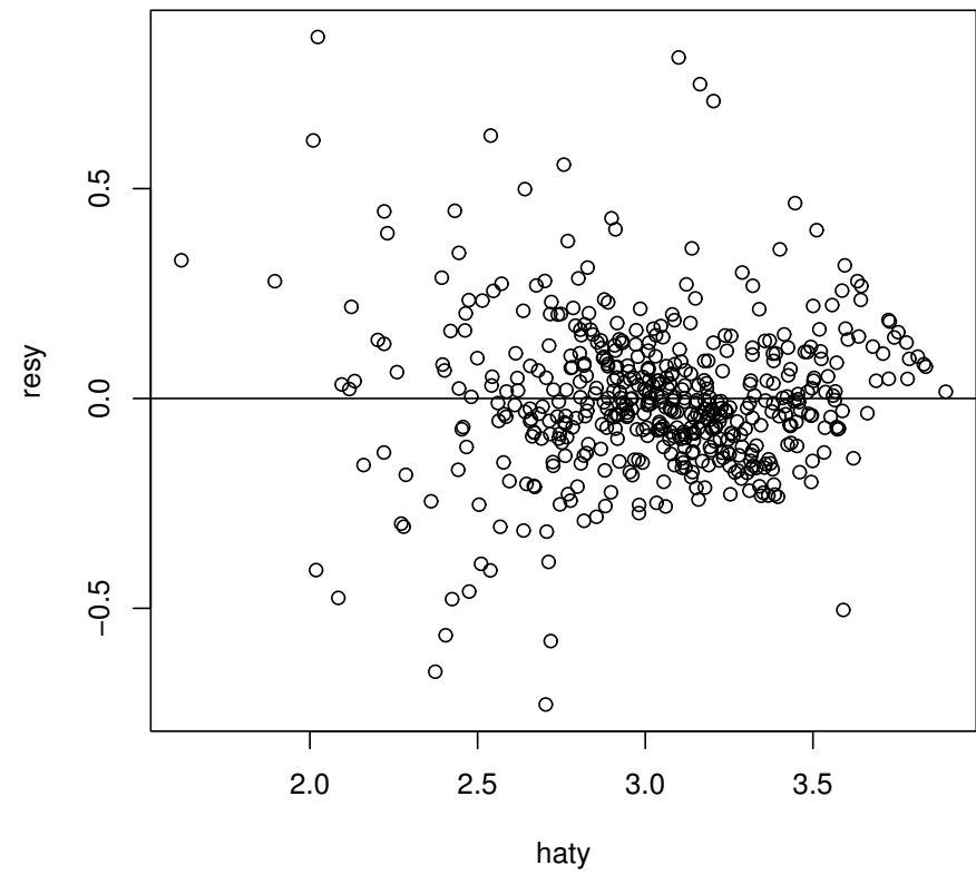
図 26 (左) (\hat{y}_t, y_t) のプロット , (右) (\hat{y}_t, e_t) のプロット
