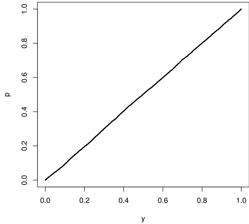
図7 (左) ヒストグラム , (右) 経験分布関数
