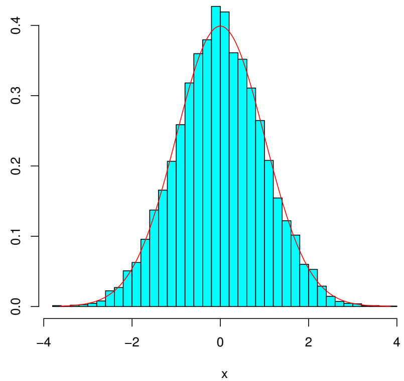
图 10 (左) 逆関数法 (指数分布), (右) 棄却法 (正規分布)
