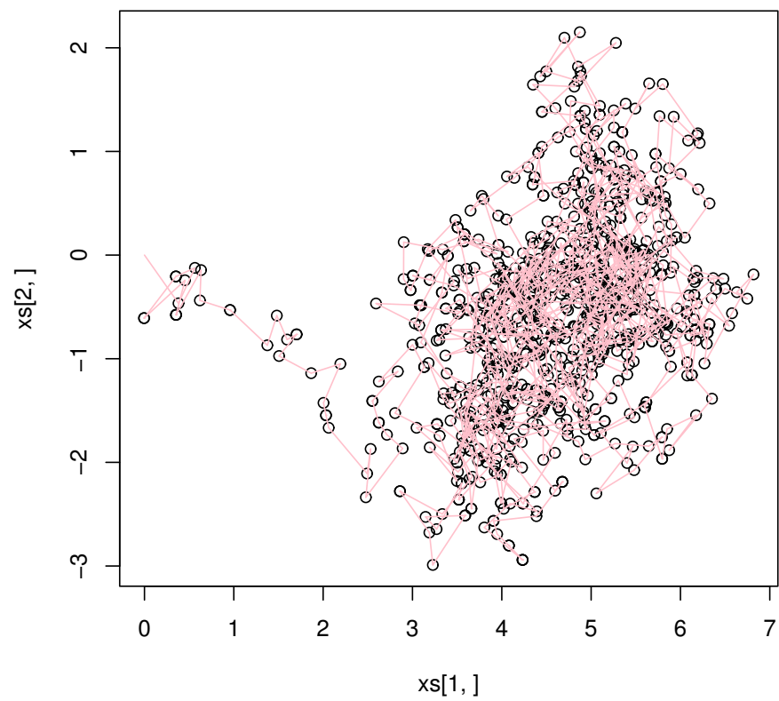
図 12 (左) 例題 1.11 の X_t , (右) \log(f(X_t))
